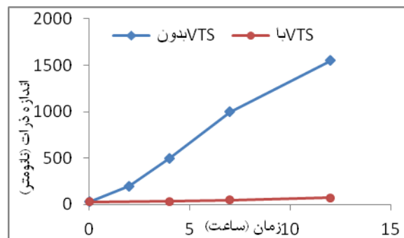
شکل ۱۷. نمودار تغییر اندازه ذرات با گذشت زمان (نمونه‌های ۶ و ۷).
