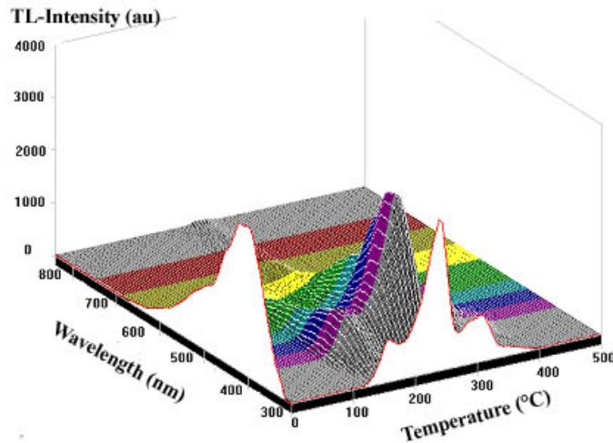
شکل ۲. طیف گرمالیانی دزیمتر LiF(Mg,Ti) بعد از پرتودهی با دز ۵۴ Gy از چشمه بتا.
