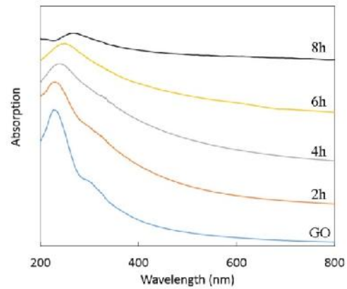
شکل ۱. (رنگی در نسخه الکترونیکی) طیف‌سنجی مرئی - فرابنفش برای اکسید گرافین و نمونه‌هایی که هر یک به مدت ۲، ۴، ۶ و ۸ ساعت تحت تابش قرار گرفته‌اند. قله واقع در طول موج ۲۲۸ نانومتر برای اکسید گرافین با افزایش زمان تابش به سمت طول موج‌های بالاتر انتقال یافته است.
