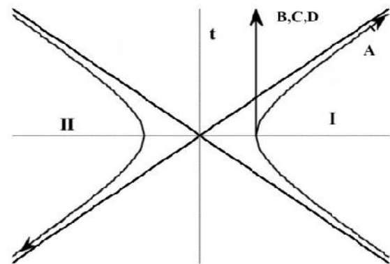
شکل ۱. دیاگرام فضای ریندلر که باب، کالین و دنی سرعت ثابتی دارند و آلیس با شتاب یکنواخت در حال حرکت می‌باشد.
