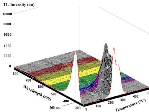
شکل ۵. (رنگی در نسخه الکترونیکی) طیف تابش LiF:Mg,Cu,P بعد از بازپخت در دمای ۴۰۰°C و پرتودهی با ۱۴Gy پرتوی بتا.
