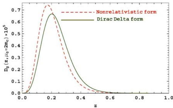
شکل ۳. (رنگی در نسخه الکترونیکی) تابع ترکش D_g^{J/\psi}(z, \mu_s = 2m_c) در مدل سوزوکی، یک بار با در نظر گرفتن تقریب تابع دلتای دیراک (۱۱) و یک بار با در نظر گرفتن تابع موج غیر نسبیته (۱۰) برای حالت مقید مزون سنگین.
