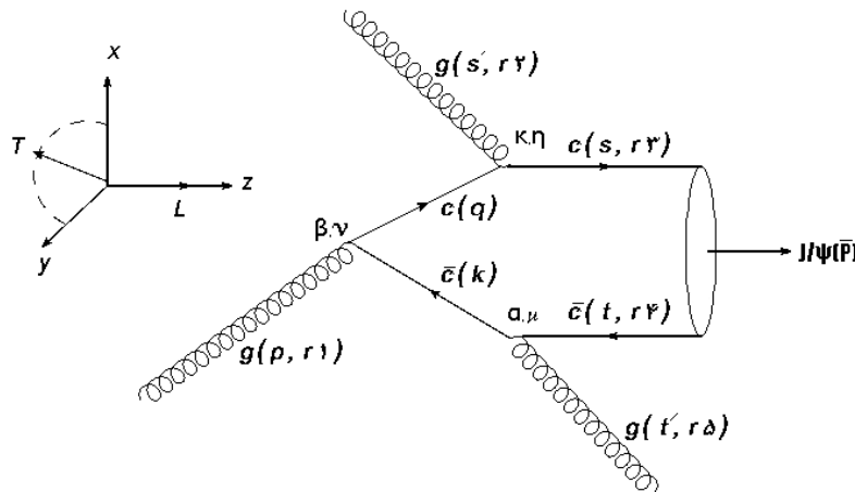
شکل ۱. نمودار فاینمن برای فرآیند ترکش g \rightarrow J/\psi + 2g در مرتبه اول اختلال. گلوئون اولیه همزمان با تشکیل حالت مقید c\bar{c} دو گلوئون نهایی منتشر می‌کند.
