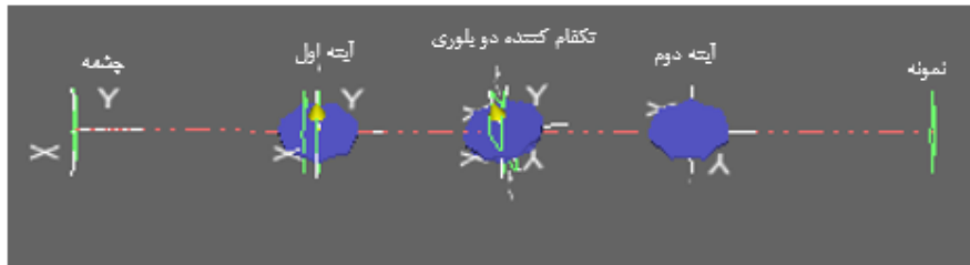
شکل ۲. تصویر شماتیک خط باریکه پراش پودری در محدوده انرژی ایکس سخت (طراحی شده با نرم افزار SHADOW) [۶ و ۷].
