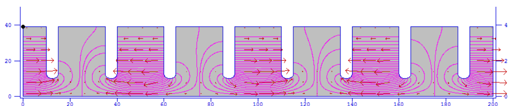
شکل ۳. شبیه‌سازی پروفایل میدان الکتریکی مد \pi/2 در نرم‌افزار سوپرفیش.
