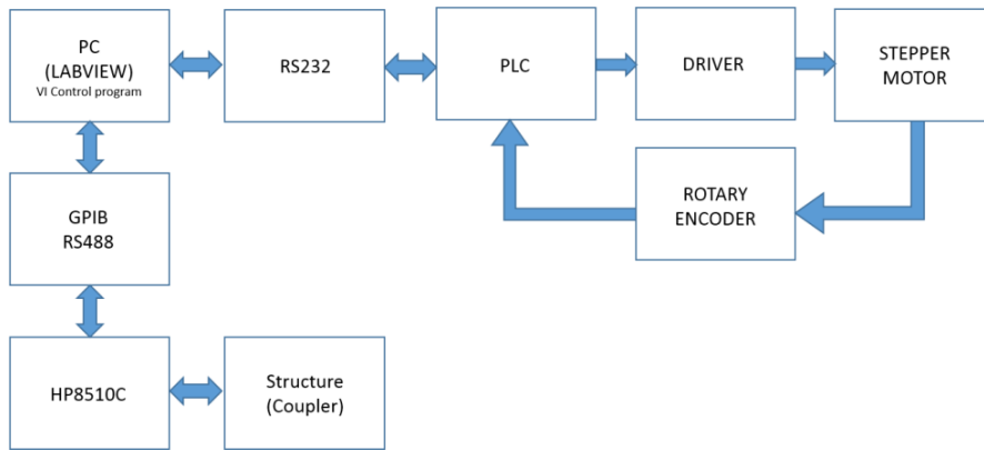
شکل ۱۱. بلوک دیاگرامی از سیستم کشش گویی.
