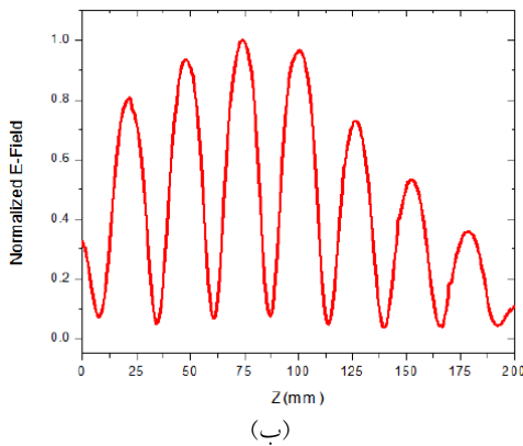
شکل ۸. پروفایل میدان الکتریکی محوری قبل از تنظیم بسامدی برای مدهای (الف) \pi/2 و (ب) \pi .
