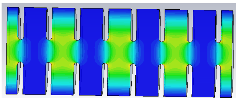
شکل ۲. شبیه‌سازی پروفایل میدان \pi/2 در نرم‌افزار CST MWS.
