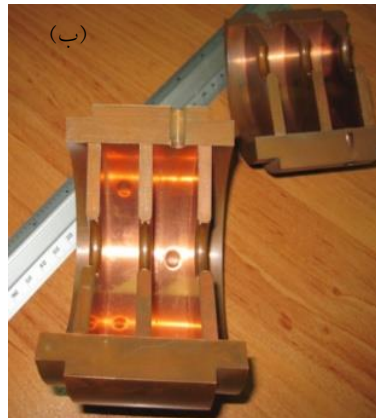
شکل ۴. (الف) ساختار ۴ سلولی ساخته شده با روش انقباضی (ب) ساختار ۴ سلولی برش زده شده با وایرکات.
