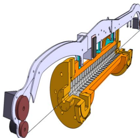
شکل ۱۰. سیستم طراحی شده برای کشش گوی.
