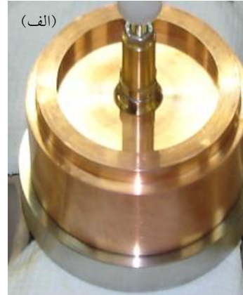
شکل ۴. (الف) ساختار ۴ سلولی ساخته شده با روش انقباضی (ب) ساختار ۴ سلولی برش زده شده با وایرکات.
