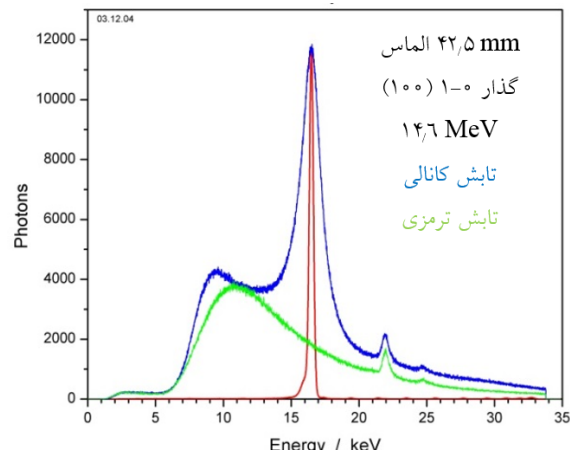
شکل ۶. طیف تابش کانالی (آبی) و تابش ترمزی (زرد) به همراه طیف تک انرژی شده با استفاده از بلور گرافیت (قرمز) از صفحه
