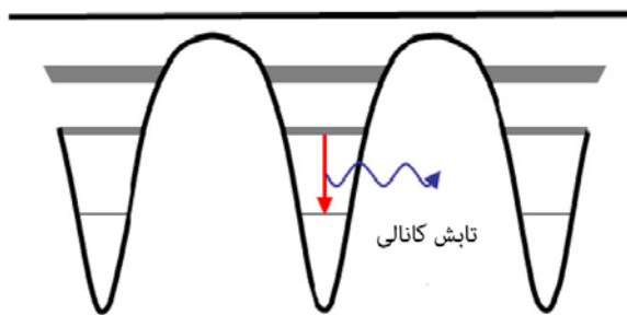
شکل ۲. توصیف کوانتمی تابش کانالی صفحه‌ای.
