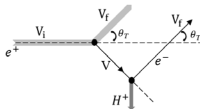
شکل ۲. نمایش سازوکار متعارف ربایش بار توماس در گذار بازچینی e^+ - H ، فرض شده است که سرعت پوزیترون منحرف شده با سرعت پوزیترونیوم تشکیل شده برابر است، جرم واسط الکترون است.
