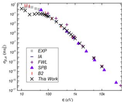
شکل ۸. (رنگی در نسخه الکترونیکی) مقایسه سطح مقطع کل تشکیل پوزیترونیم پایه بر حسب انرژی در کانال ورودی حاصل از روش (۱) و CC (x) با سایر روش‌ها □ از منبع [۱۲] و [۱۳]، - از منبع [۱۴]، + از منبع [۱۵]، Δ از منبع [۱۶]، | از منبع [۱۷].
