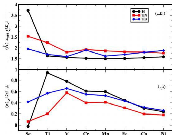
شکل ۲. (رنگی در نسخه الکترونیکی) (الف) ارتفاع بهینه شده اتم‌های 3d -TM از سطح BN (صفحه XY ) را در سه وضعیت H, TN و TB بر حسب آنگستروم نشان می‌دهد. (ب) مقدار بار انتقالی از اتم‌های 3d -TM به زیر سطح H-BN 2D را بر حسب واحد بار الکترون نمایش می‌دهد. در این شکل نتایج مربوط به ساختارهای H, TN و TB به ترتیب با دایره و رنگ مشکی، مربع و رنگ قرمز و لوزی با رنگ آبی مشخص شده‌اند.
