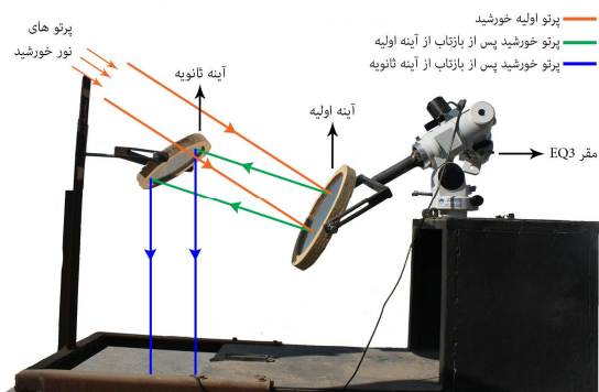
شکل ۲. (رنگی در نسخه الکترونیکی) نمای کلی سیستم اپتیکی و مقر.
