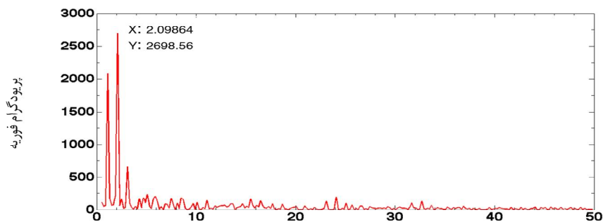
شکل ۸. (رنگی در نسخه الکترونیکی) پریودگرام فوریه برای سری زمانی XZ Dra . بسامد (روز -۱ )
