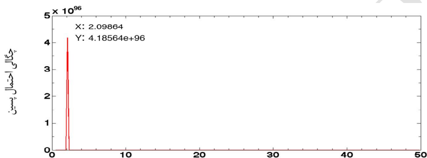
شکل ۹. (رنگی در نسخه الکترونیکی) چگالی احتمال بسین بسامد برای سری زمانی XZ Dra . بسامد (روز -۱ )
