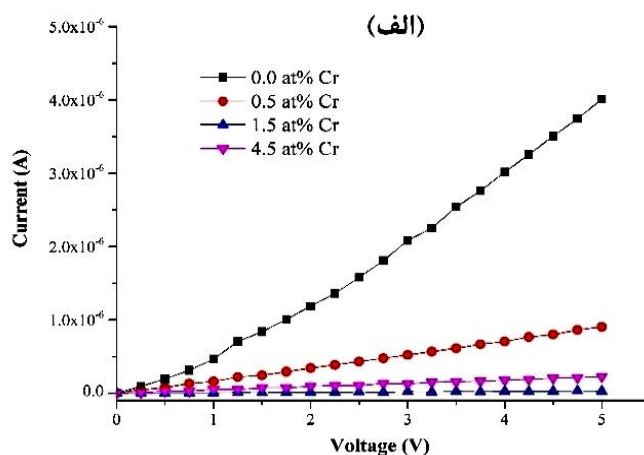
شکل ۴. (رنگی در نسخه الکترونیکی) نمودارهای I-V حسگر نانومیله اکسید روی.
