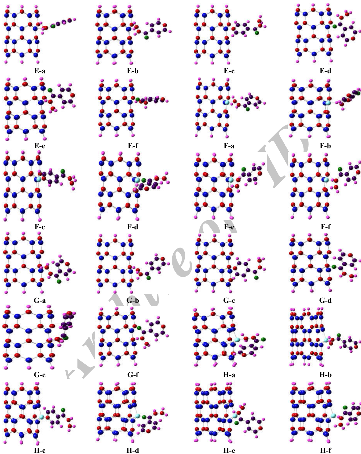
شکل ۱. (رنگی در نسخه الکترونیکی) ساختارهای بهینه شده جذب ایزونیازید بر روی سطح نانولوله گالیم نیتريد خالص و جایگزین شده برای مدل‌های E, F, H.G.
