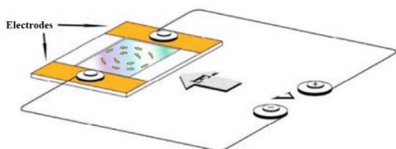
شکل ۱. (رنگی در نسخه الکترونیکی) نمایی از چیدمان مورد استفاده جهت چرخش نانوسیال.
