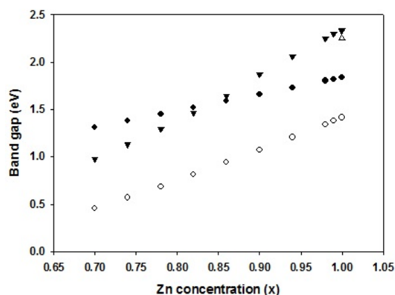
شکل ۲. گاف انرژی ترکیب سه تایی ZHT با استفاده از تقریب GGA بدون برهم کنش اسپین-مدار (دایره توخالی)، تقریب GGA حضور برهم کنش اسپین-مدار (دایره توپر) و در نهایت تقریب GW (مثلث توپر). مقدار تجربی گاف انرژی ZnTe با مثلث تو خالی آمده است، که نشانگر درستی محاسبات گاف انرژی با تقریب GW است.
