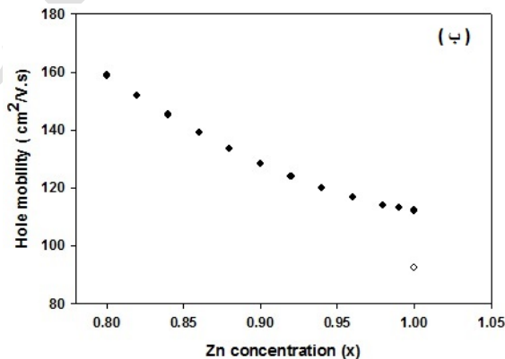
شکل ۴. تحرک‌پذیری (الف) الکترون‌ها و (ب) حفره‌ها در ترکیب سه‌تایی ZHT. در شکل (الف) مقدار تجربی تحرک‌پذیری الکترون با مثلث توپر و در شکل (ب) مقدار تجربی تحرک‌پذیری حفره‌ها با دایره توخالی نشان داده شده است.
