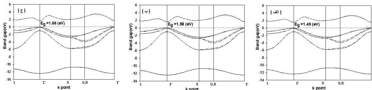
شکل ۳. نوار انرژی ترکیب سه‌تایی ZHT، (الف) x=0.8 ، (ب) x=0.85 ، (ج) x=0.9 که مستقیم بودن گاف را نشان می‌دهد.
