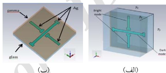
شکل ۲. (رنگی در نسخه الکترونیکی) یاخته واحد سه بعدی فراماده.
