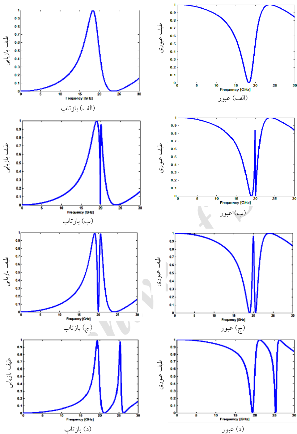
شکل ۸. (رنگی در نسخه الکترونیکی) طیف عبوری و بازتاب ساختار، (الف) حالت متقارن، (ب) به ازای L_p = 2.75 \text{ mm} ، (ج) L_p = 3 \text{ mm} ، (د) L_p = 3.25 \text{ mm} .
