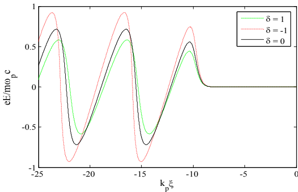
شکل ۱. (رنگی در نسخه الکترونیکی) دامنه بی بعد شده میدان عقبه طولی برای پالسی با a_0 = 1 و k_p \xi_c = -20 و پلاسما بی با n_p = 1.09 \times 10^{18} \text{ cm}^{-3} بر حسب k_p \xi_c ، خط نقطه \sigma = -1 ، خط چین \sigma = 1 و خط پیوسته \sigma = 0 .
