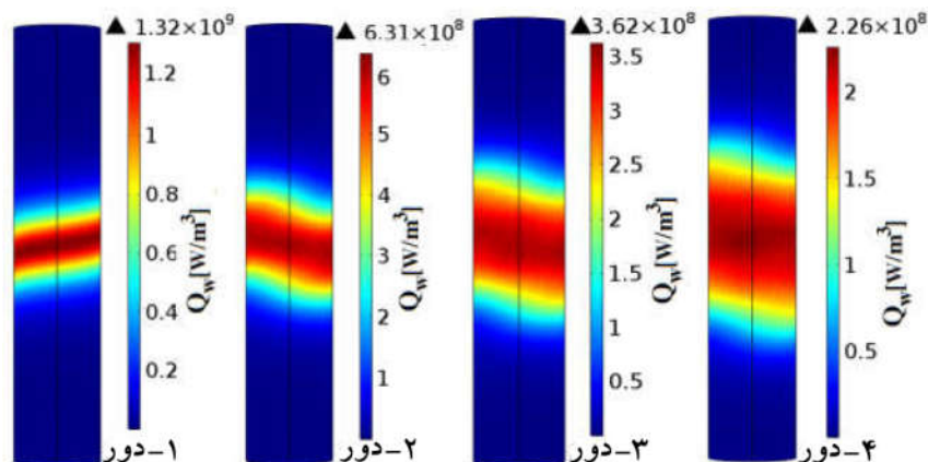
شکل ۹. (رنگی در نسخه الکترونیکی) توزیع و شدت گرمای تولید شده در قطعه کار برای پیچ‌های ۱، ۲، ۳ و ۴ حلقه‌ای.
