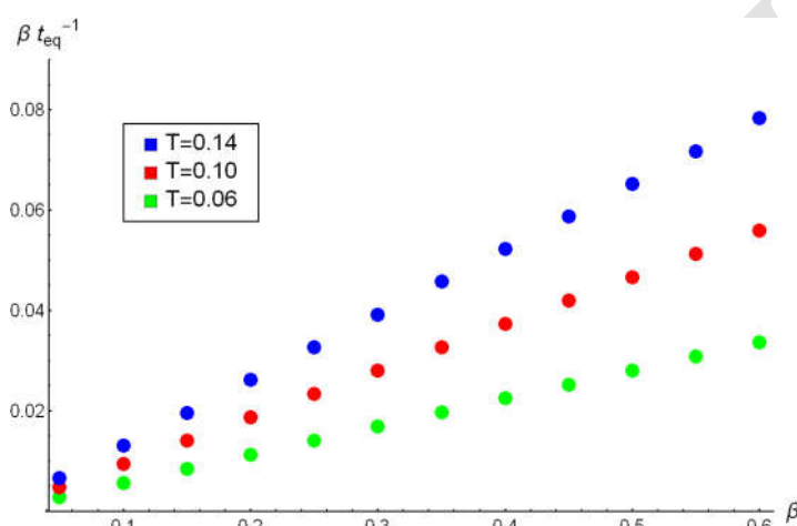
شکل ۲. \beta t_{eq}^{-1} بر حسب مقادیر مختلف سرعت تزریق انرژی.
