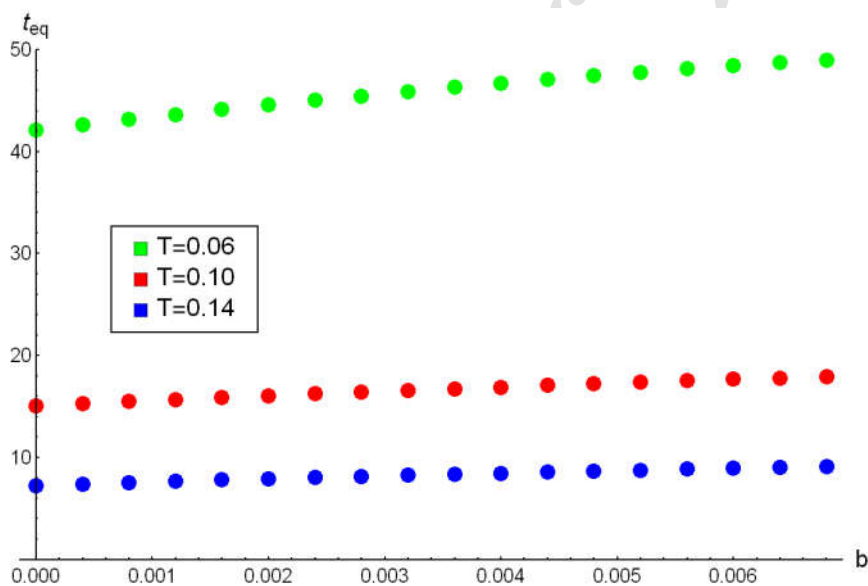
شکل ۴. زمان تعادل بر حسب ضریب تصحیحات ثابت جفت‌شدگی برای \Delta = 2 .
