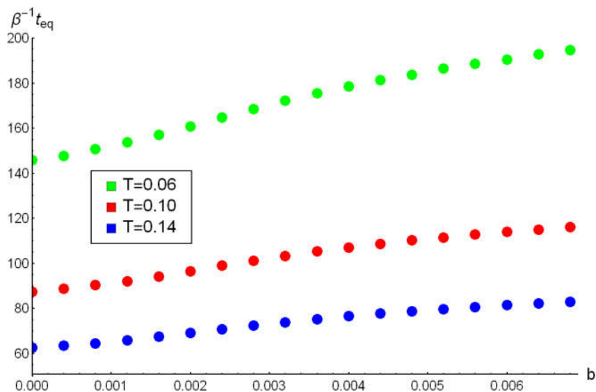
شکل ۳. کمیت \beta^{-1}t_{eq} بر حسب بزرگی ضریب تصحیحات ثابت جفت‌شدگی b برای \Delta = 3 .
