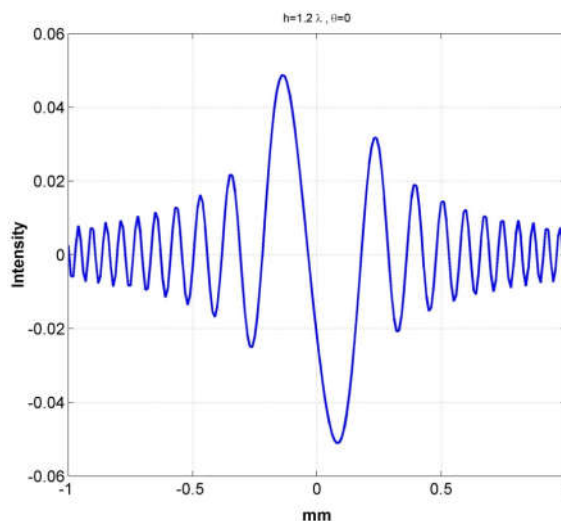
شکل ۲. (رنگی در نسخه الکترونیکی) توزیع شدت برای پراش فرنل از پله ای به ارتفاع 1/2\lambda و فرود عمودی.
