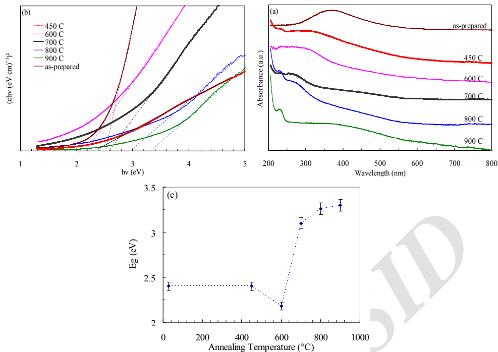
شکل ۱. (رنگی در نسخه الکترونیکی) (a) جذب و (b) ترسیم تاک طیف اکسید گرافین آراسته شده با دی‌اکسید تیتانیوم در ناحیه مرئی - فرابنفش نمونه‌ها بلافاصله پس از ساخت و پخت شده در پنج دمای مختلف، (c) گاف نواری اپتیکی به دست آمده از ترسیم تاک نمونه‌های پخت شده برحسب دمای پخت.
