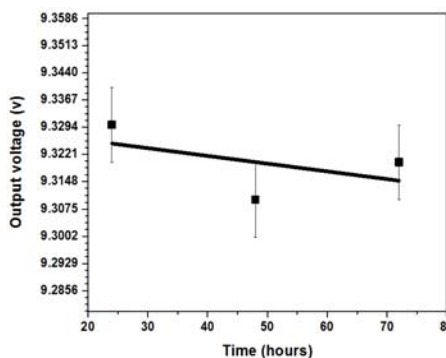
شکل ۶. نمودار پایداری زمانی حسگر.
