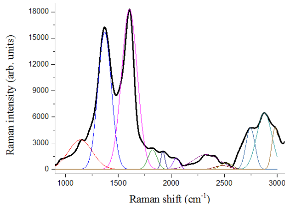
شکل ۵. (رنگی در نسخه الکترونیکی) واپیچش طیف رامان GO، به دست آمده با ۵۳۲ نانومتر.
