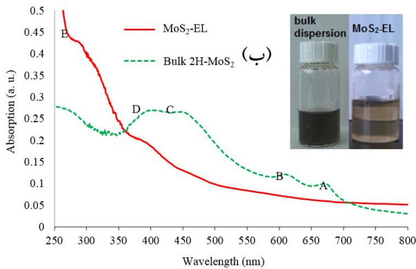
شکل ۳. (رنگی در نسخه الکترونیکی) طیف جذب اپتیکی نانوصفحات سنتز شده: (الف) نمونه WS ۲ -EL و (ب) نمونه MoS ۲ -EL. طیف جذب اپتیکی استاندارد توده ۲ WS ۲ -2H و MoS ۲ -2H مربوط به هر نمودار نیز برای مقایسه رسم شده است. در گوشه هر نمودار، تصویر نمونه‌های سنتز شده و سوسپانسیون ماده توده قبل از سنتز مربوط به هر ماده نشان داده شده است.
