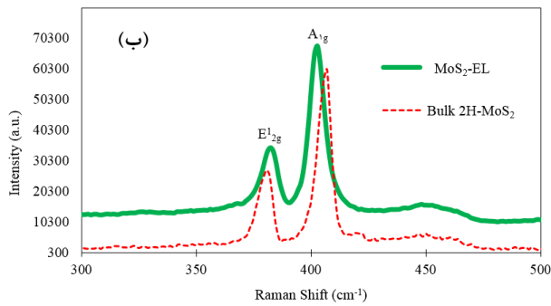
شکل ۶. (رنگی در نسخه الکترونیکی) طیف رامان نانوصفحات سنتز شده: (الف) نمونه WS_2 -EL و (ب) نمونه MoS_2 -EL. طیف رامان استاندارد توده 2H-WS_2 و 2H-MoS_2 نیز در هر نمودار برای مقایسه، رسم شده است.
