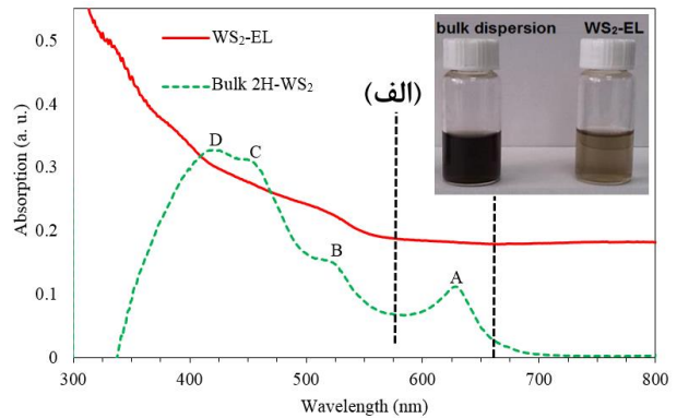
شکل ۳. (رنگی در نسخه الکترونیکی) طیف جذب اپتیکی نانوصفحات سنتز شده: (الف) نمونه WS ۲ -EL و (ب) نمونه MoS ۲ -EL. طیف جذب اپتیکی استاندارد توده ۲ WS ۲ -2H و MoS ۲ -2H مربوط به هر نمودار نیز برای مقایسه رسم شده است. در گوشه هر نمودار، تصویر نمونه‌های سنتز شده و سوسپانسیون ماده توده قبل از سنتز مربوط به هر ماده نشان داده شده است.
