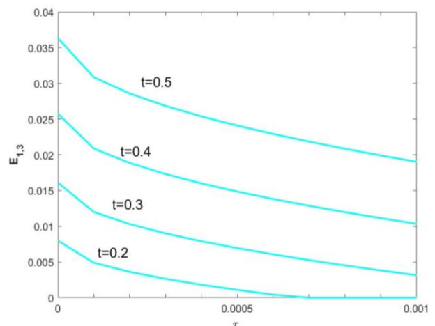
شکل ۴. (رنگی در نسخه الکترونیکی) در هم تنیدگی بین کیوبیت اول و سوم بر حسب دما در زمان‌های مختلف، وقتی حالت اولیه شامل یک برانگیختگی در کیوبیت اول است.
