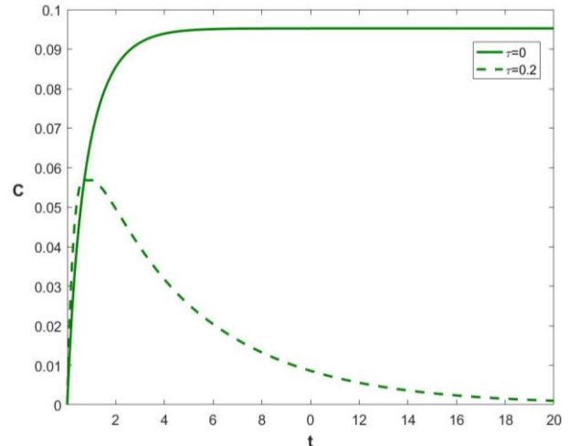
شکل ۶. (رنگی در نسخه الکترونیکی) میزان همدوسی کوانتومی در سیستم بر حسب زمان. منحنی توپر مربوط به حالتی است که دمای محیط صفر است، و \tau = 0 ، و منحنی خط چین نشان دهنده میزان همدوسی در \tau = 0.2 است.
