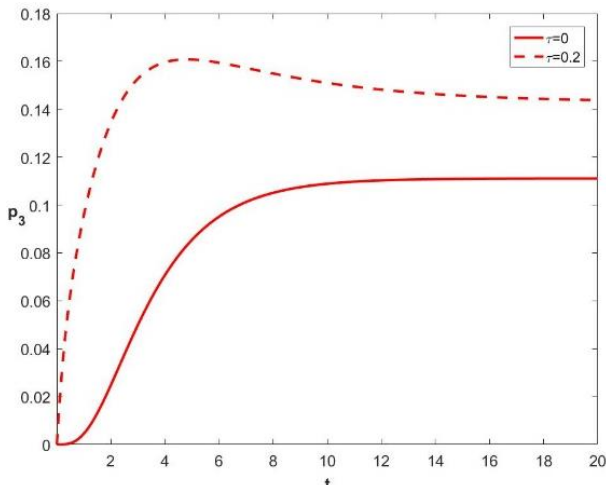
شکل ۷. (رنگی در نسخه الکترونیکی) احتمال این که کیوبیت آخر در حالت برانگیخته باشد بر حسب زمان. منحنی توپر مربوط به حالتی است که دمای محیط صفر است و منحنی خط چین مربوط به محیط در دمای غیر صفر و \tau = 0.2 است.
