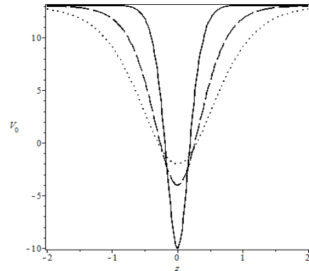
شکل ۱. پتانسیل مؤثر میدان اسپینوری الکو به ازای p = 0.5 (منحنی خطی)، p = 1 (منحنی خط چین) و p = 1.5 (منحنی نقطه چین) و H = 2 و M_{\text{Elko}} = 1 .
