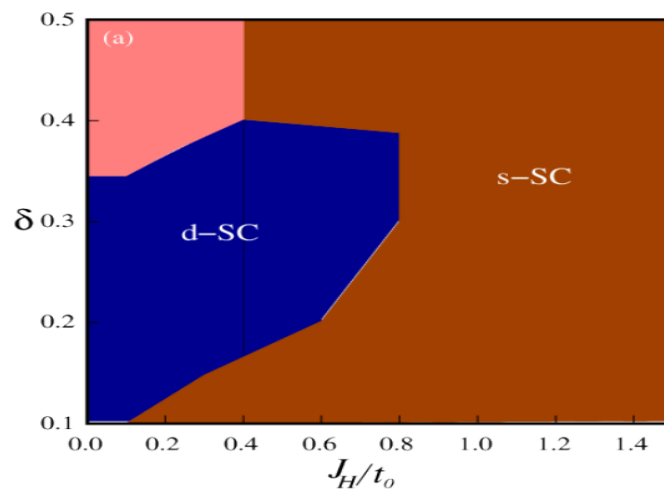
شکل ۴. (رنگی در نسخه الکترونیکی) سیمای فاز ابررسانایی مدل کیتائو-هایزنبرگ گسترده با برهم‌کنش‌های تبادلی در مقیاس K = -\Gamma = t_0 با استفاده از روش میدان میانگین به عنوان تابعی از برهم‌کنش هایزنبرگ پادرومغناطیس ( J_H > 0 ) در واحد انتگرال پرش ( t_0 ) و مقدار آلابدگی ( \delta ).
