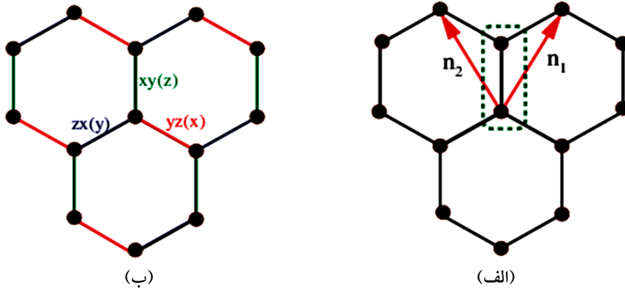
شکل ۱. (رنگی در نسخه الکترونیکی) (الف) هندسه شبکه لانه زنبوری در فضای حقیقی با یاخته واحد دو اتمی با بردارهای اصلی \vec{n}_1 و \vec{n}_2 را نشان می‌دهد و (ب) هر جایگاه از طریق سه پیوند غیرمعادل به نزدیک‌ترین همسایه‌اش روی شبکه لانه زنبوری متصل شده است. رنگ‌های قرمز، آبی و سبز به ترتیب پیوندهای \alpha\beta(\gamma) = yz(x), zx(y), xy(z) را مشخص می‌کنند که \beta, \alpha و \gamma مؤلفه‌های اسپین برهم‌کنشی مربوطه به هر پیوند را نشان می‌دهند.
