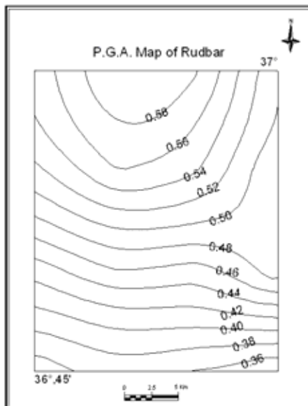
شکل ۹- نقشه بیشینه شتاب زلزله در منطقه مورد مطالعه
