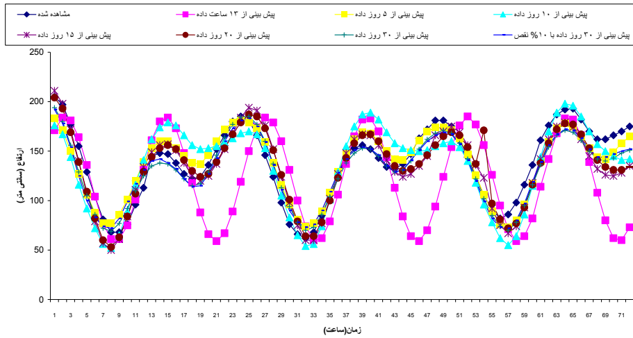
نمودار ۱- نمودار داده‌های اصلی و نیز پیش‌بینی‌های انجام شده در بوشهر.
