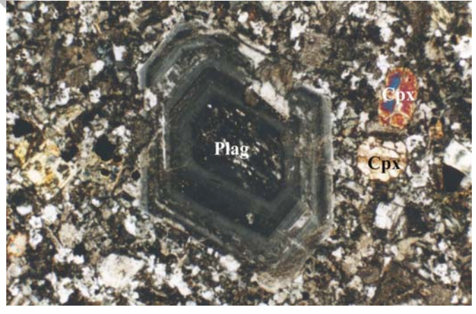
:Cpx : Plag
