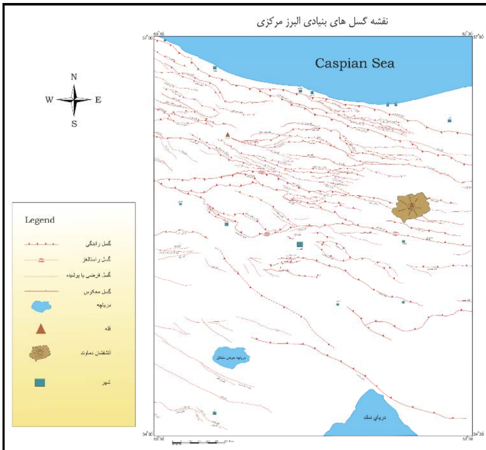
شکل ۷: نقشه گسل‌های بنیادی منطقه با طول بیش از ۲۰ کیلومتر (تهیه شده براساس نقشه های زمین شناسی ۱/۱۰۰۰۰۰ و ۱/۲۵۰۰۰۰ منطقه)
