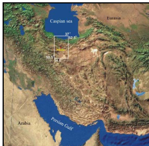
شکل ۵: محدوده مورد بررسی در روی مدل ارتفاعی رقومی (DEM) فلات ایران (Google Earth).
