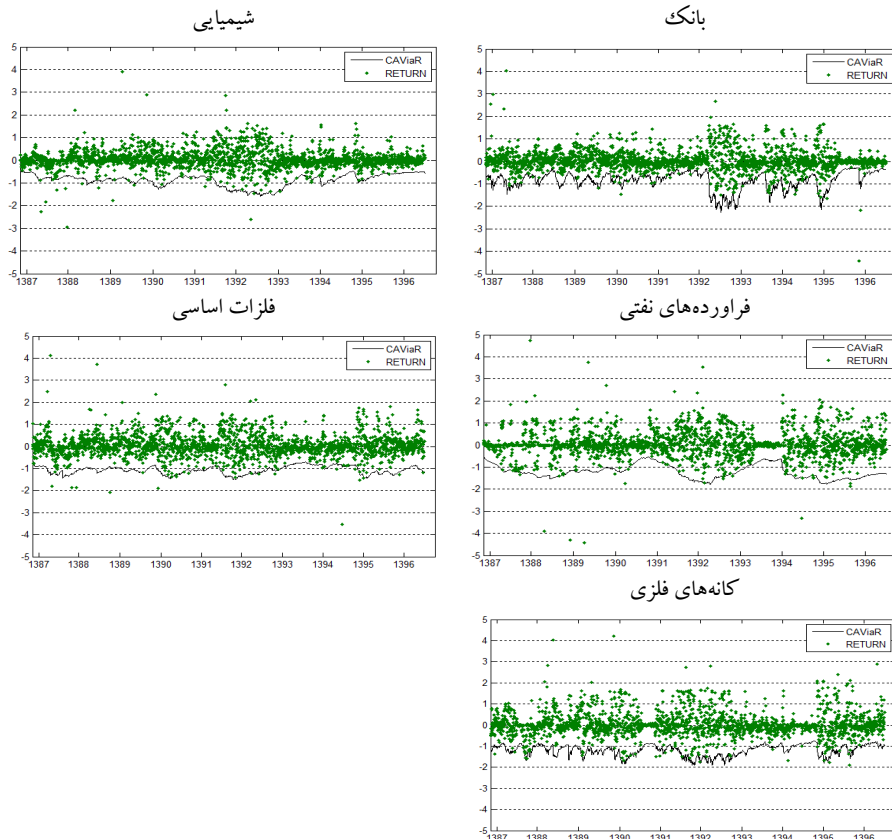
نمودار ۳- CAViaR صنایع منتخب در سطح ۰.۱٪ چندک با استفاده از روش VAR for VaR
