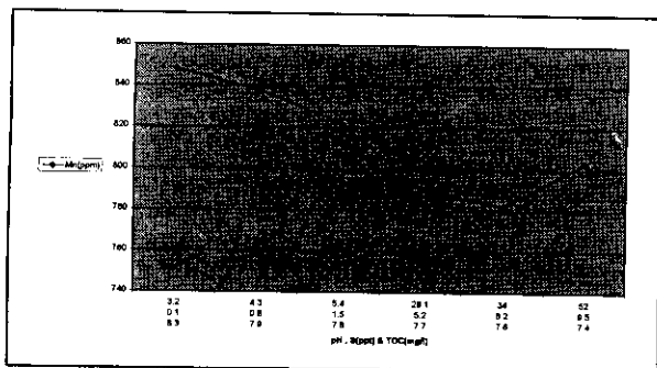
شکل شماره (۵): تغییرات غلظت منگنز در رسوبات نسبت به pH، TOC و شوری در حین اختلاط با آب دریا
