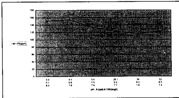
شکل شماره (۱۱): تغییرات غلظت سرب در ذرات معلق نسبت به pH، TOC، و شوری در حین اختلاط با آب دریا
