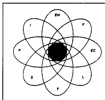
شکل (۱): نمودار Venn
