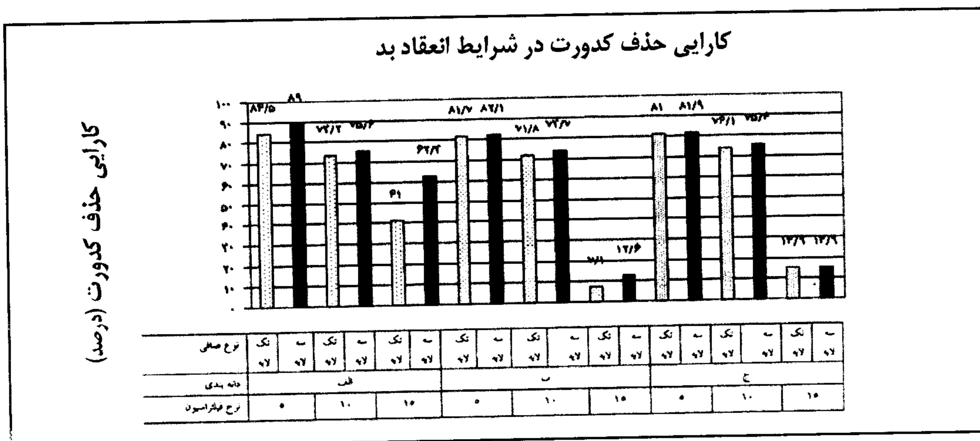
شکل شماره (۴): کارایی حذف کدورت در شرایط انعقاد بد بدون تزریق کلرورفریک
