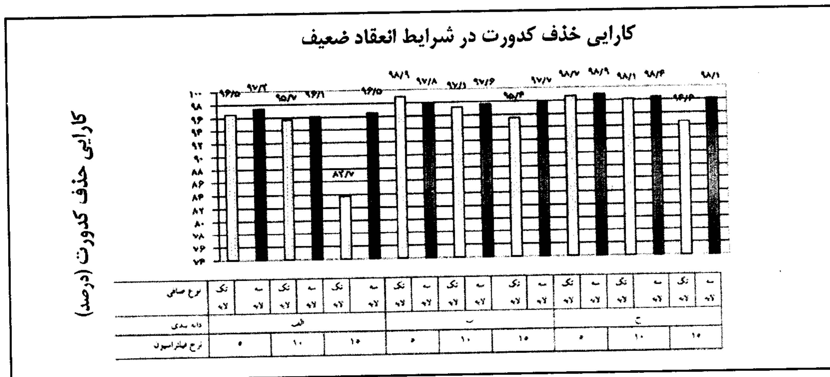
شکل شماره (۳): کارایی حذف کدورت در شرایط انعقاد ضعیف با تزریق ۱/۵ میلی گرم در لیتر کلرورفریک
