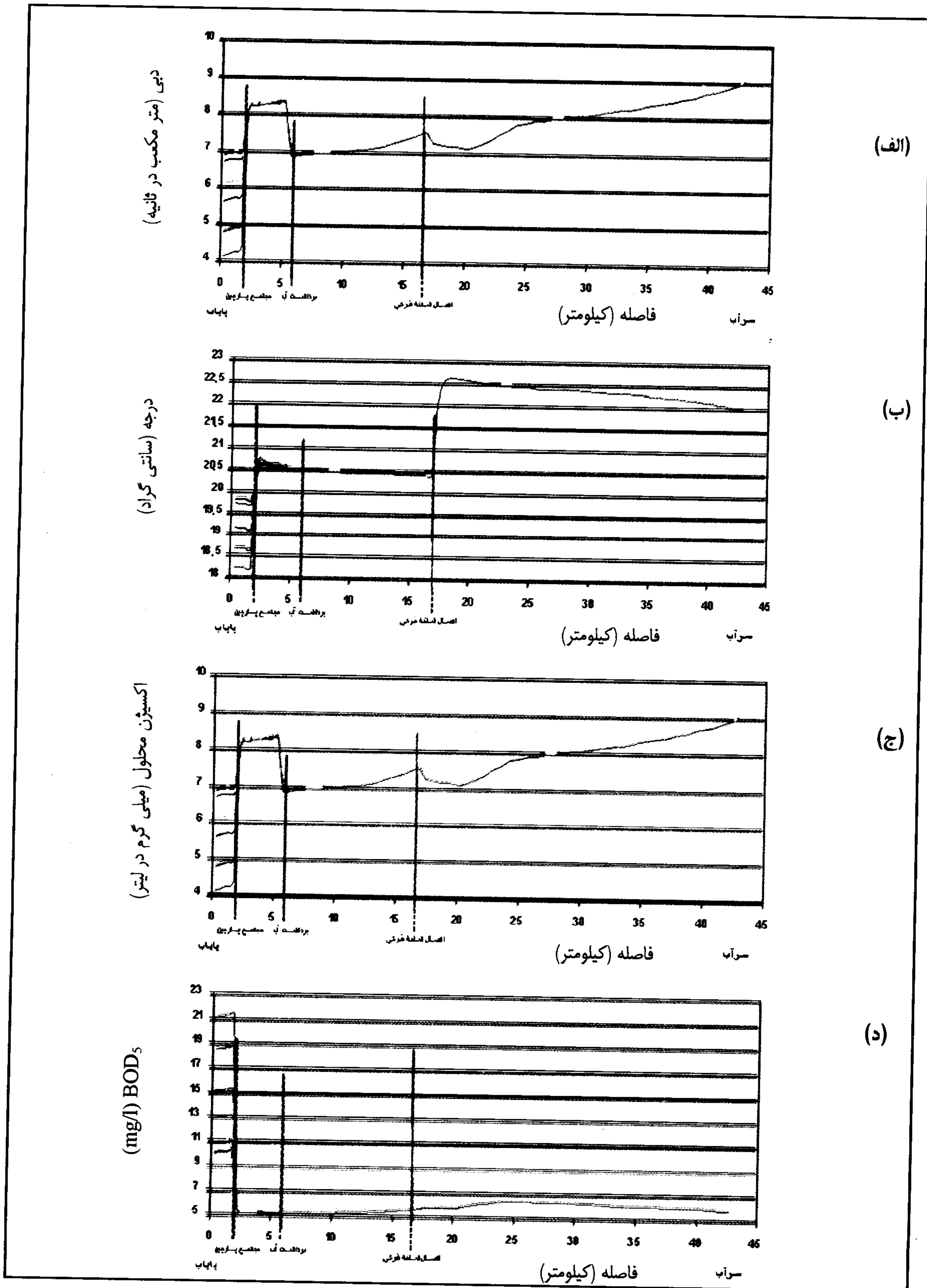
شکل (۲) تغییرات (الف) دبی، (ب) درجه حرارت، (ج) غلظت اکسیژن محلول و (د) اکسیژن خواهی پنج روزه در طول شاخه اصلی رودخانه در تیرماه به ازای ۱، ۲، ۳، ۴، ۵ و ۵ متر مکعب در ثانیه برداشت آب.
