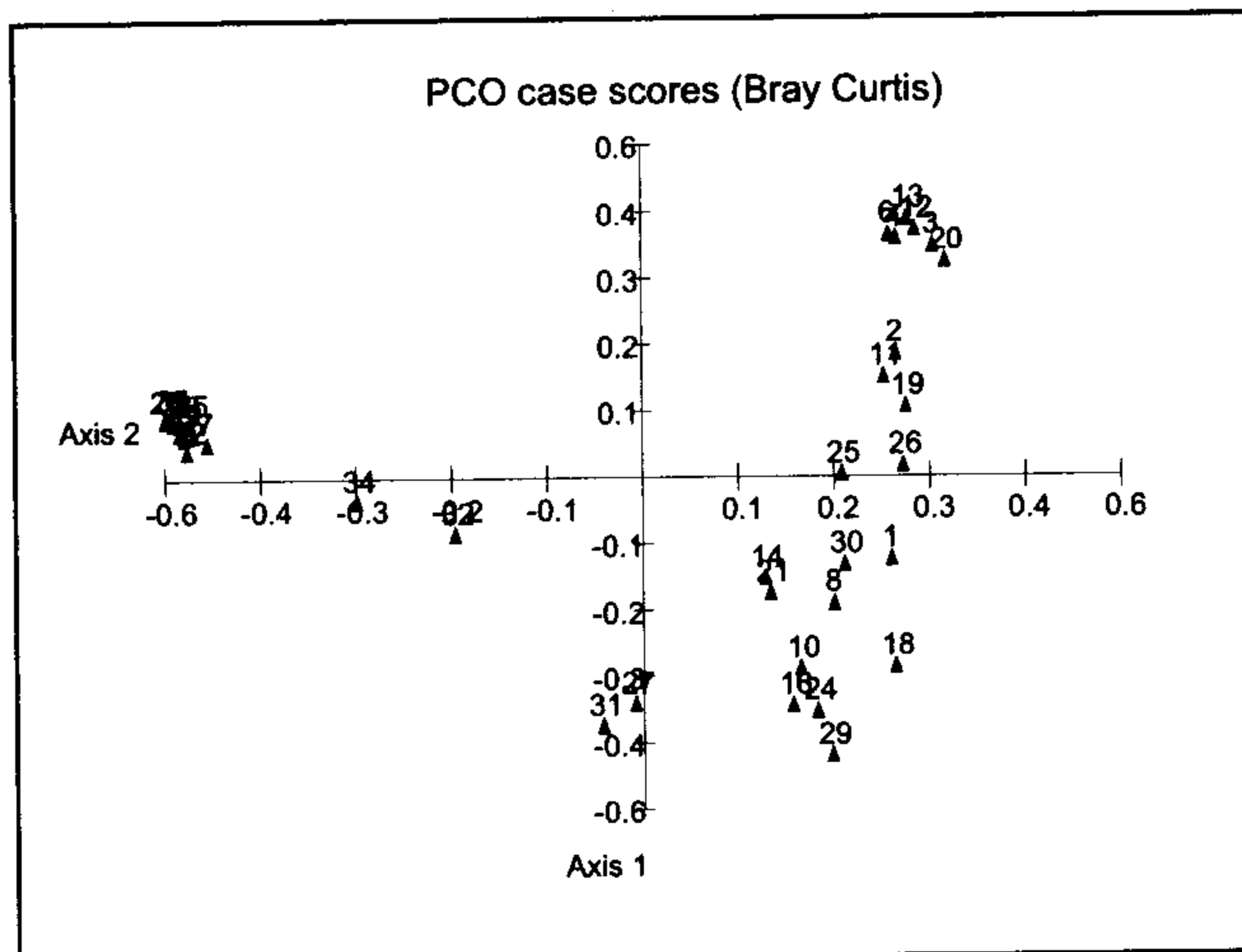
شکل شماره (۳): تفکیک توده ها روی محورهای اوردیناسیون
