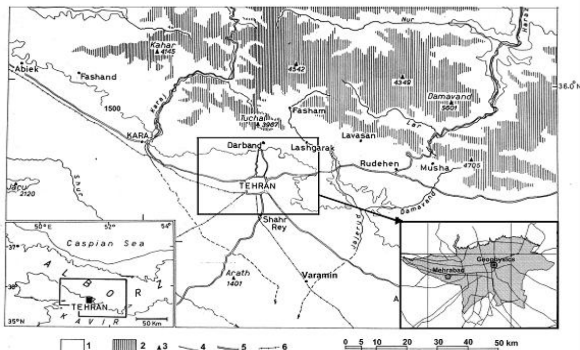
شکل شماره (۶): موقعیت جغرافیایی ایستگاه هواشناسی مؤسسه ژئوفیزیک دانشگاه تهران و دامنه کوههای البرز واقع در شمال تهران (شماره‌های ۱ تا ۶ به ترتیب معرف ۱: مناطق با ارتفاع کمتر از ۱۵۰۰ متر از سطح دریا، ۲: مناطق با ارتفاع کمتر از ۳۰۰۰ متر، ۳: قله‌های کوه، ۴: رودخانه‌ها، ۵: بزرگراهها و ۶: خطوط راه آهن هستند).
