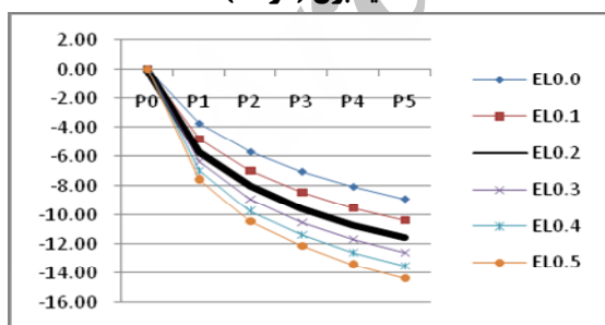
نمودار شماره (۱۰): تغییر در انتشار CO 2 با سناریوهای کاهش در لایه فسیلی (درصد)
