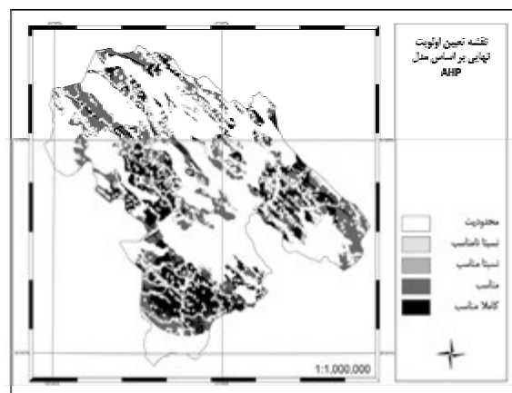
شکل شماره (۵): نقشه تعیین اولویت نهایی بر اساس مدل AHP
