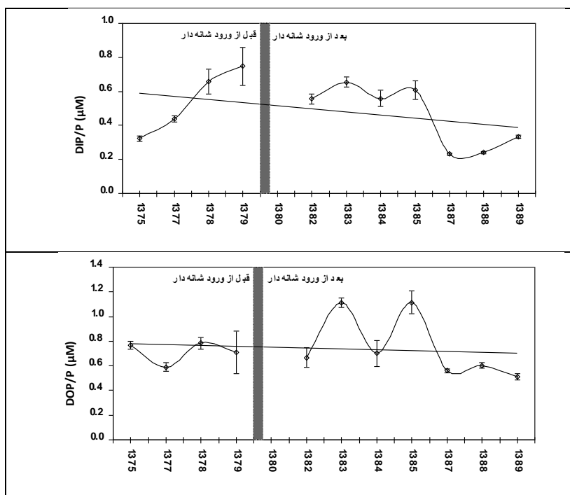
نمودار ۲. میانگین تغییرات فسفر معدنی (µM، DIP) و آلی (µM، DOP) همراه خط روند در سال‌های مختلف حوزه جنوبی دریای خزر
