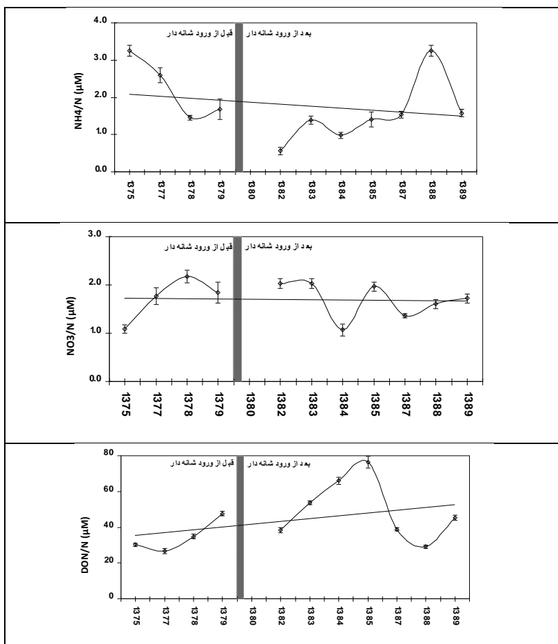
نمودار ۱. میانگین تغییرات ازت آمونیومی (µM، NH 4 )، نیتراتی (µM، NO 3 ) و آلی (µM، DON) همراه خط روند در سال‌های مختلف حوزه جنوبی دریای خزر
