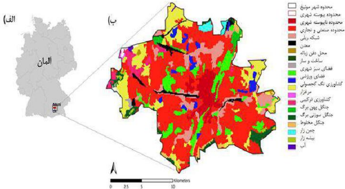
شکل ۲. نقشه پوشش زمینی و پراکنش آن‌ها در محدوده مورد مطالعه: الف) محدوده مورد مطالعه به رنگ قرمز مشخص شده است؛ ب) نقشه کاربری زمینی با ۲۱ گروه
