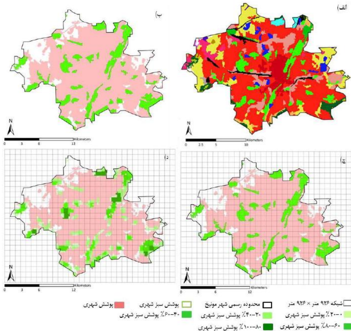
شکل ۴. الف) نقشه کاربری کورین منطقه مورد مطالعه؛ ب) نقشه طبقه‌بندی مجدد شده و همگن از محدوده مورد مطالعه؛ ج) ماتریسی از میزان حضور کاربری زمین (پوشش شهری و پوشش سبز شهری) در هر پیکسل از سنجنده مودیس؛ د) نقشه درصد حضور پوشش سبز شهری در هر پیکسل.
