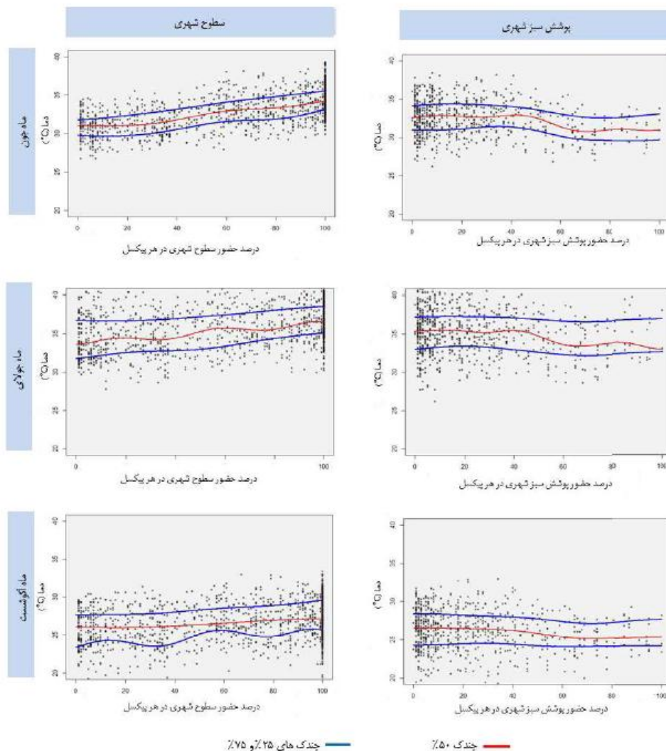
شکل ۵. رابطه بین دمای سطحی یا میزان گستردگی کاربری زمین (سطوح شهری یا پوشش گیاهی) در هر پیکسل را نشان می‌دهد نمودار مربوط به دمای سطحی ماه‌های گرم سال ۲۰۰۶ است.
