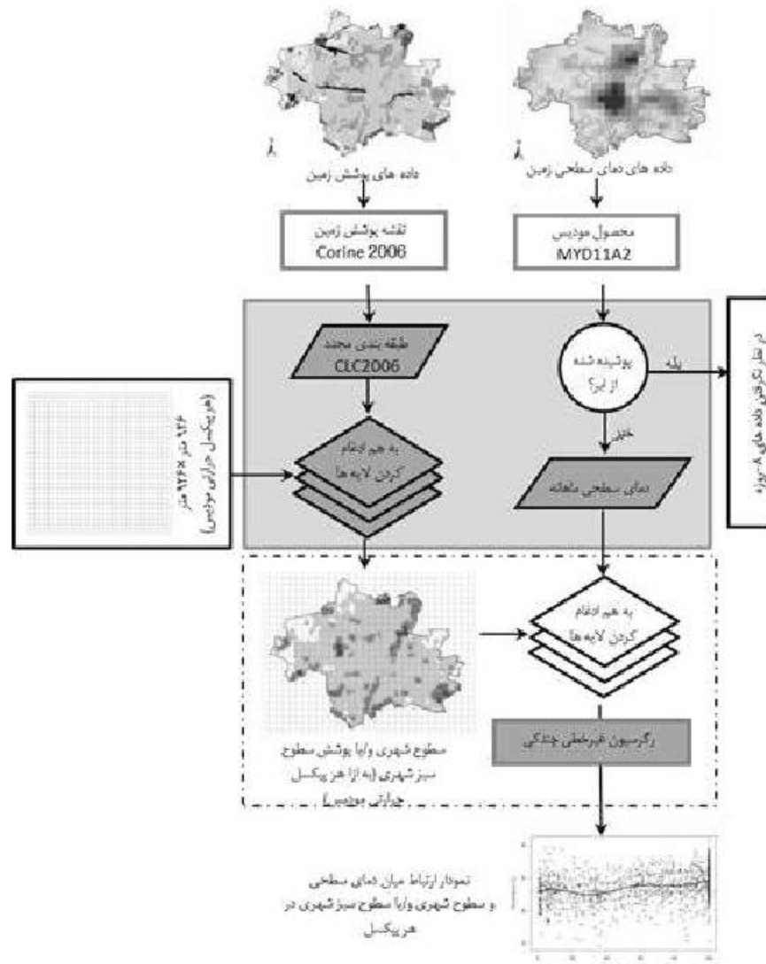
شکل ۱. نمودار روند کلی این مطالعه
