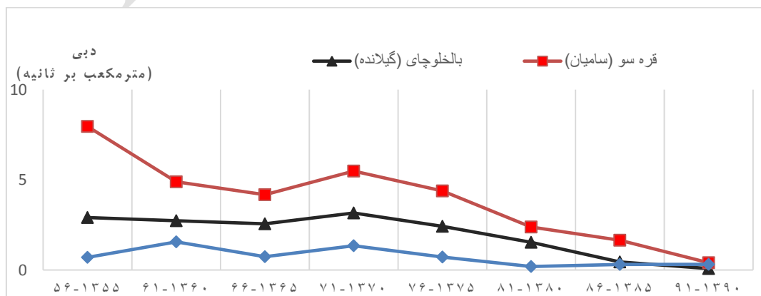
شکل ۱۱. روند میانگین سالانه دبی رودخانه بالخلوچای (ایستگاه گیلانده)، رودخانه قوری‌چای (ایستگاه کوره تپلاق) و رودخانه قره‌سو (ایستگاه سامیان)
