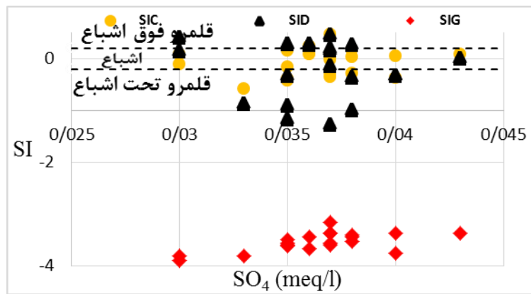
شکل ۸. نمایه‌های اشباع کلسیت، دولومیت و ژپس نمونه‌های منطقه مورد مطالعه
