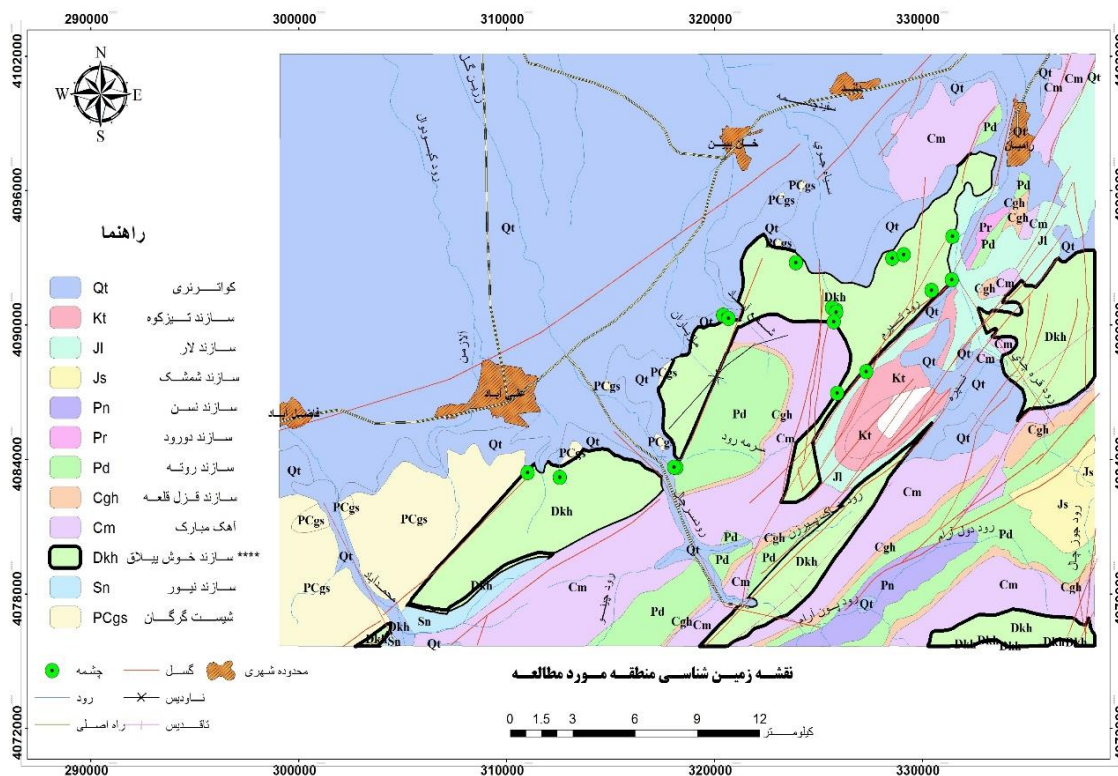
شکل ۱. نقشه موقعیت مکانی و زمین‌شناسی منطقه مورد مطالعه
