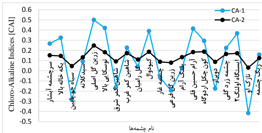
شکل ۶. نمایه Chloro-Alkaline ۵ نمونه های آب منطقه مورد مطالعه
