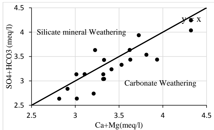
شکل ۴. طرح پراکنده نشان دهنده نقش نسبی هوازدگی سنگهای سیلیکاته و کربناته در هیدروژمی آب
