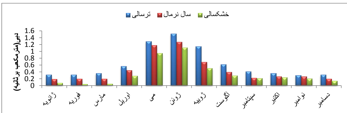
شکل ۴. سری زمانی ماهانه جریان (شکل بالا: دلیچای، شکل پایین: نرم)
