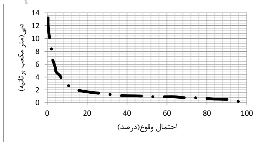
شکل ۳. منحنی تداوم جریان (بالا: الرم، پایین: دلچجای)
