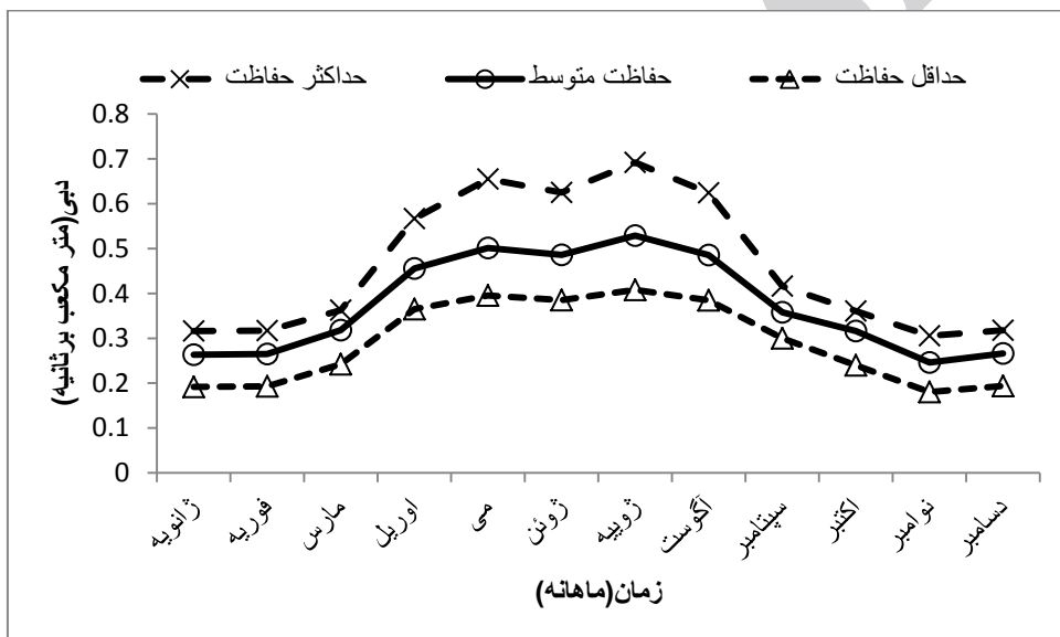
شکل ۸. رژیم جریان اکولوژیک پیشنهادی (شکل بالا: دلچای، شکل پایین: الرم)
