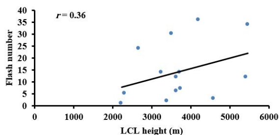
شکل ۲. تغییرات تعداد درخت آذرخش با ارتفاع LCL در ایستگاه مهرآباد تهران در طی سال‌های ۲۰۰۹ تا ۲۰۱۳ با استفاده از داده‌های LIS
