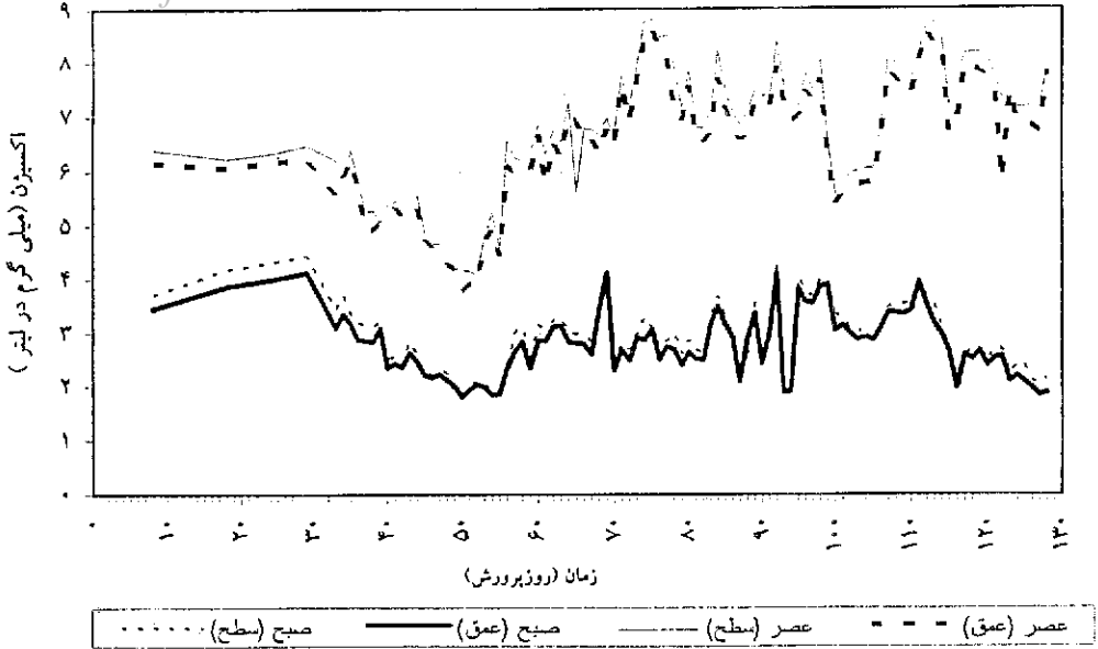
نمودار ۳: تغییرات اکسیژن در استخر شماره ۲ زراستی در طول دوره پرورش (۱۳۷۸)
