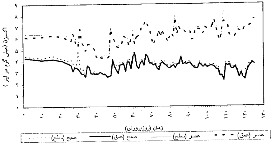
نمودار ۷: تغییرات اکسیژن در استخر شماره ۱۲ مزرعه مه‌کیش در طول دوره پرورش (۱۳۷۸)
