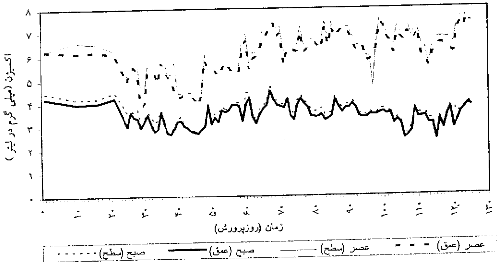
نمودار ۶: تغییرات اکسیژن در استخر شماره ۴ مزرعه اداره کار در طول دوره پرورش (۱۳۷۸)
