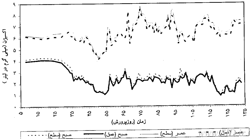
۴۴ نمودار ۸: تغییرات اکسیژن در استخر شماره ۱۳ مزرعه مه‌کیش در طول دوره پرورش (۱۳۷۸)
