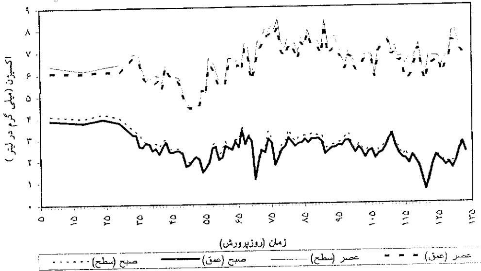
نمودار ۵: تغییرات اکسیژن در استخر شماره ۳ مزرعه اداره کار در طول دوره پرورش (۱۳۷۸)
