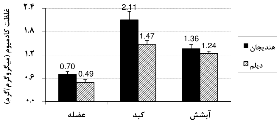
نمودار ۱: میانگین غلظت کادمیوم در بافت آبشش، کبد و عضله ماهیان منطقه هندیجان و دیلم در فصل تابستان ۱۳۸۷. بارها نمایانگر انحراف استاندارد می‌باشند.
